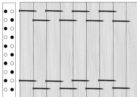
Figura N° 7 DIAGRAMA CONFIGURACIÓN NLT
