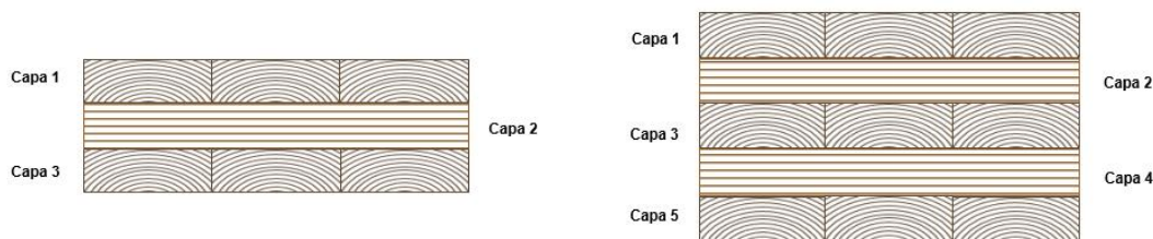
Figura N° 2 CONFIGURACIÓN DEL PANEL CLT PARA 3 Y 5 CAPAS
