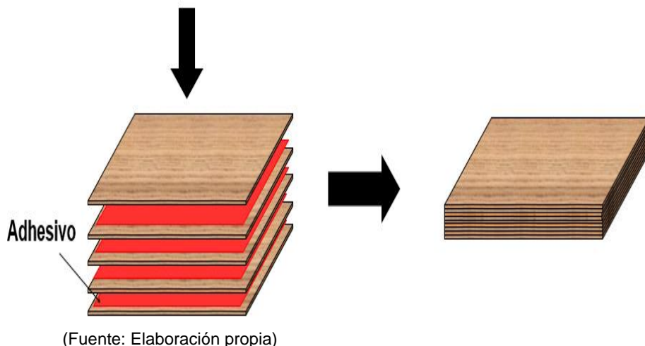
Figura N° 4 DIAGRAMA DE CONFIGURACIÓN LVL
