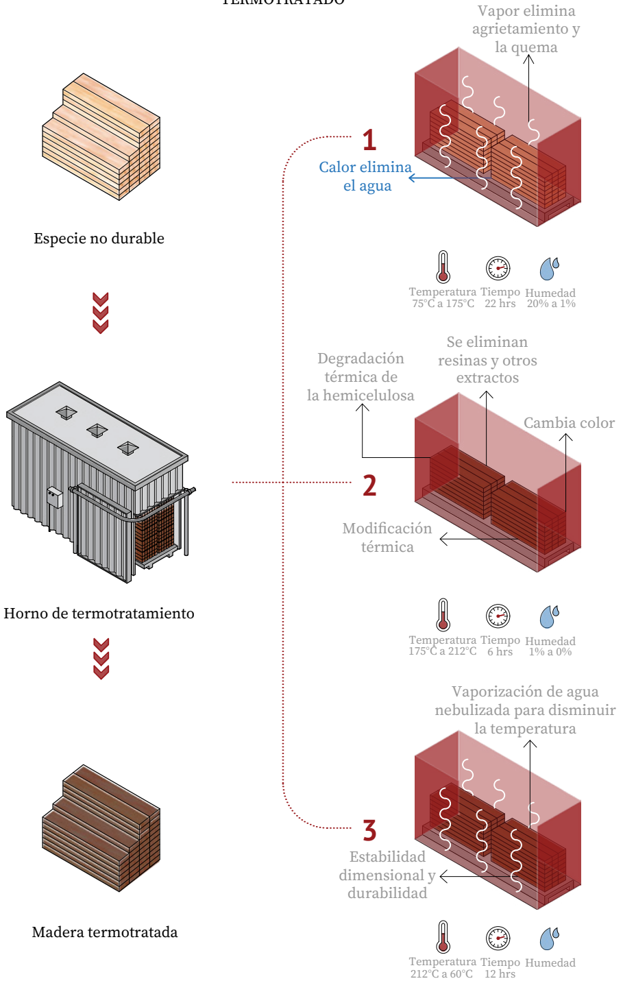
Figura 5.15 – Proceso Madera termotratado
