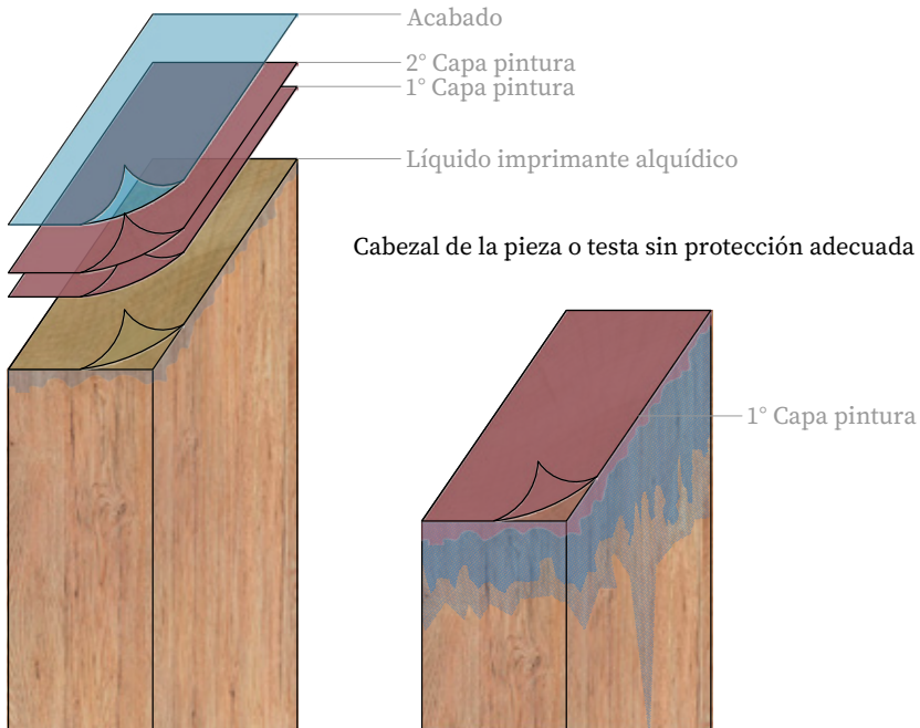
Figura 4.16 – Protección en la testa o cabezal de la pieza
