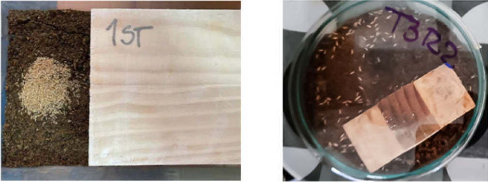
Figura 3.16 – Instalación de probetas para ensayo frente a termitas
