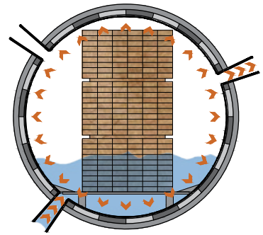
2. Inundación Ingresa la solución preservante mientras se mantiene el vacío
