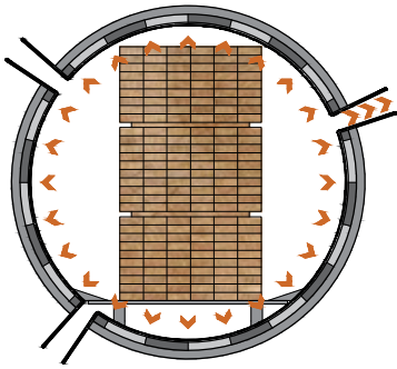
1. Vacío inicial Para eliminar el aire de las células de la madera
