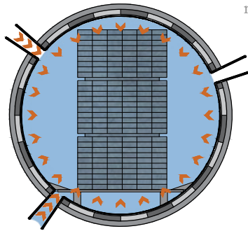
3. Presión Se libera el vacío y se aplica presión para introducir la solución a la madera
